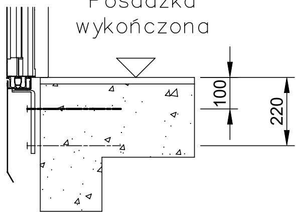
Szczegół A
